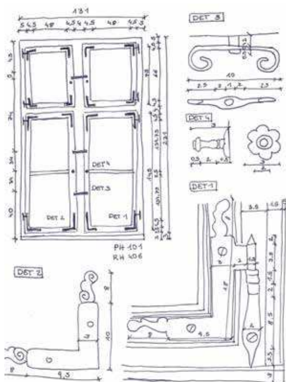
Abb.28: Detaillierte Maßskizzen zur Dokumentation eines Fensters in der Herrengasse 16.
